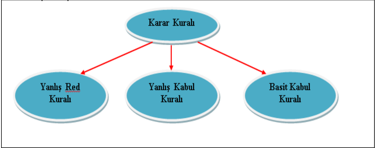
Şekil 1 : Karar Kuralı
